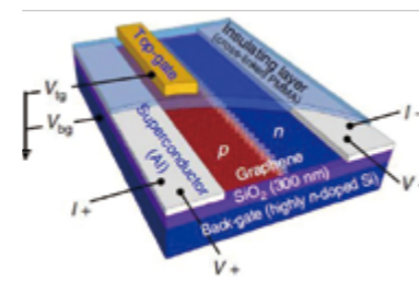
그래핀을 이용한 초전류 트랜지스터의 구성도
