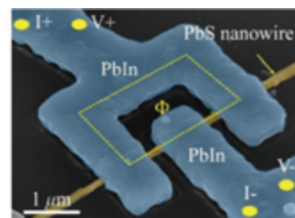
반도체 나노선을 이용한 초전류 양자 간섭 소자의 전자현미경 사진
